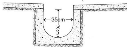
U型排水渠橫切面圖
